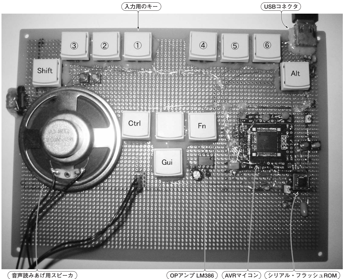
写真1 文字を音声で読み上げるUSB点字キーボード
