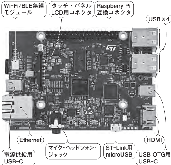
(a) 表面 (LCDの下側) にはRaspberry Pi互換コネクタ
