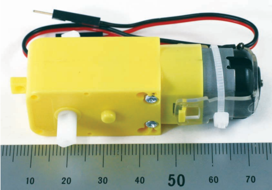
写真1 1個数百円で入手可能な小型でギヤ付きでトルクが出せる通称「TTモータ」
