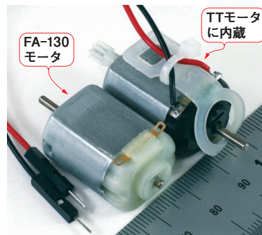
写真2 TTモータに付いているモータとFA-130モータの比較
