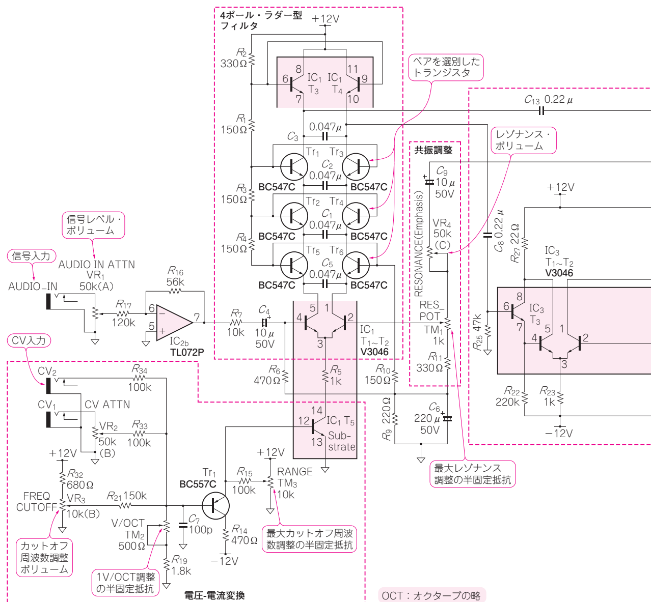
図1 製作した電子楽器用のラダー型電圧制御フィルタVCF回路 MiniMoog (Moog) を参考にした
