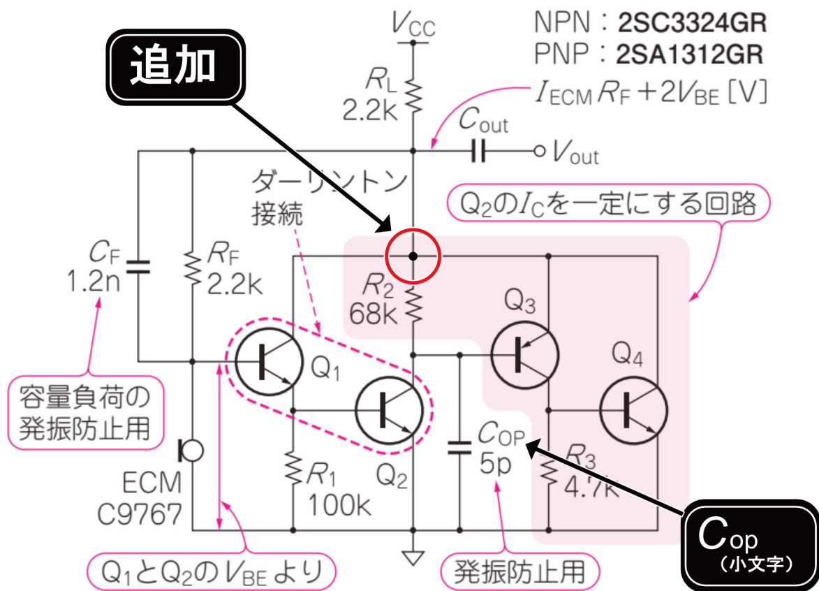
図9 SR-TIAのトランジスタ4石タイプ
