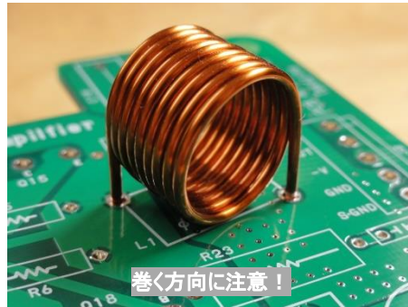
太さ13~14mmのボールペンに巻く
