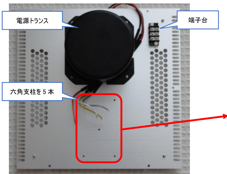
「電源トランス」「端子台」を固定
