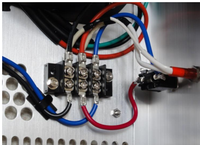
端子台は全て丸端子処理
