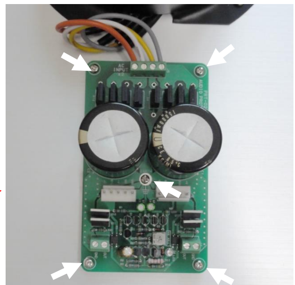
電源基板を固定
