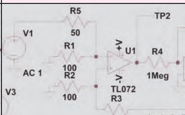
測定回路
