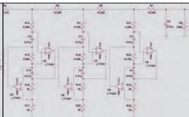
フィルタ回路
