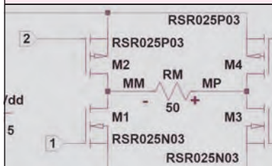
モータ駆動回路
