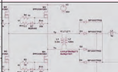
電源回路
