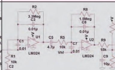
センサ回路
