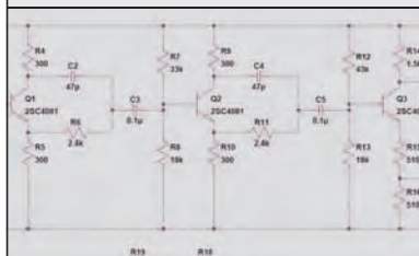
発振回路
