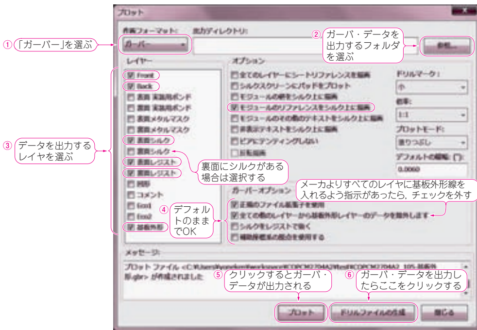
図2 手順1：発注に必要なデータの一つ「ガーバ・データ」を出力する「プロット画面」
