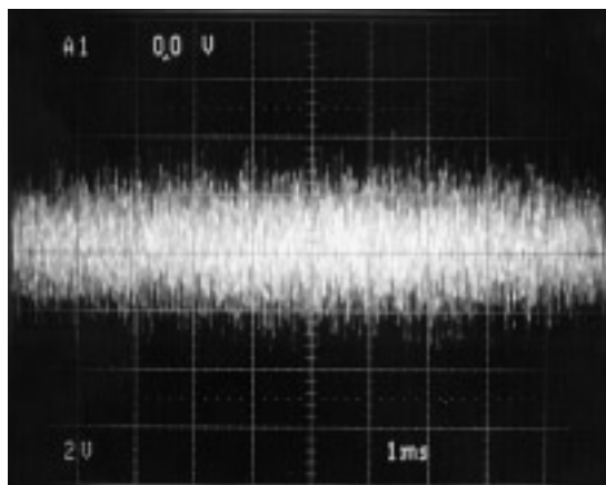
(b) 上限周波数100 kHz(-3 dB), 1 V RMS
