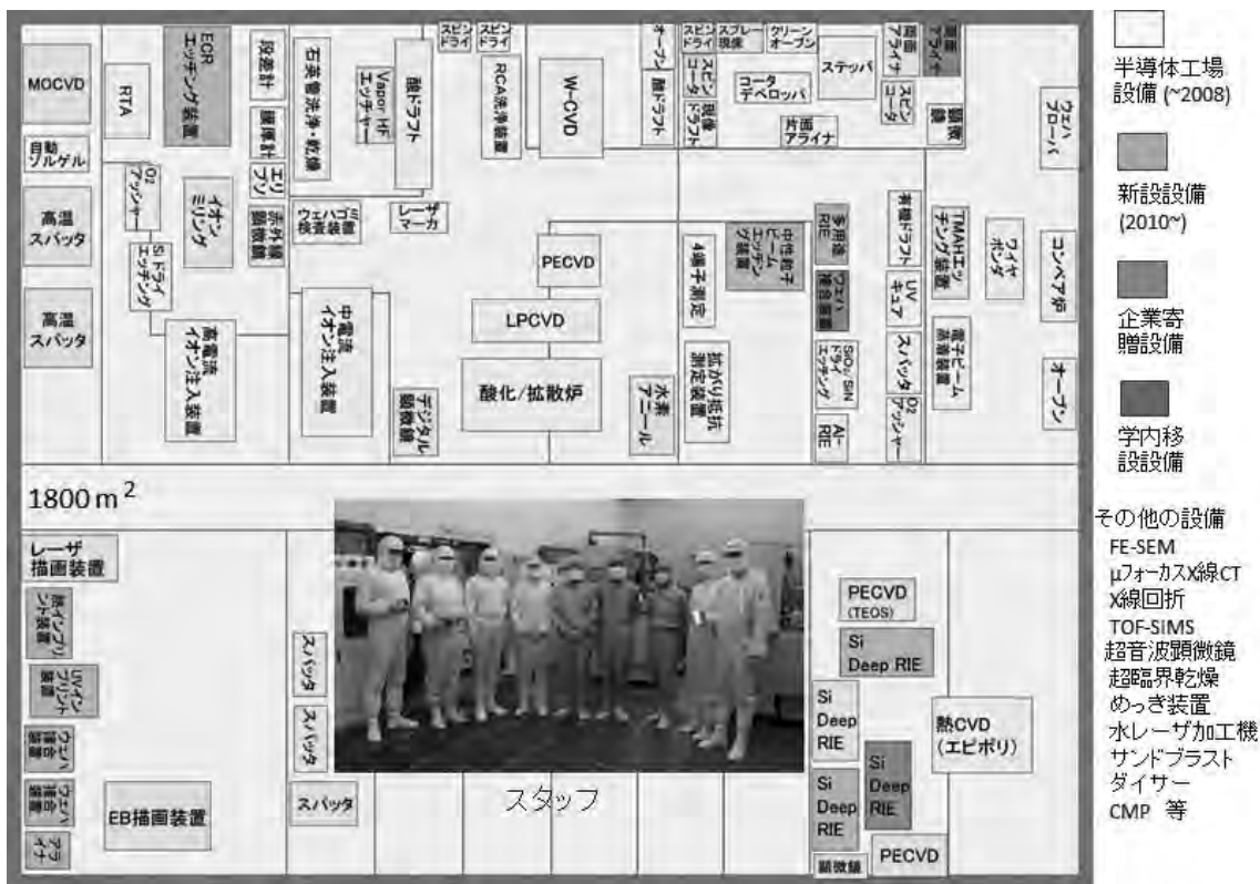
(a) クリーン・ルーム (1800m 2 ) のレイアウト
