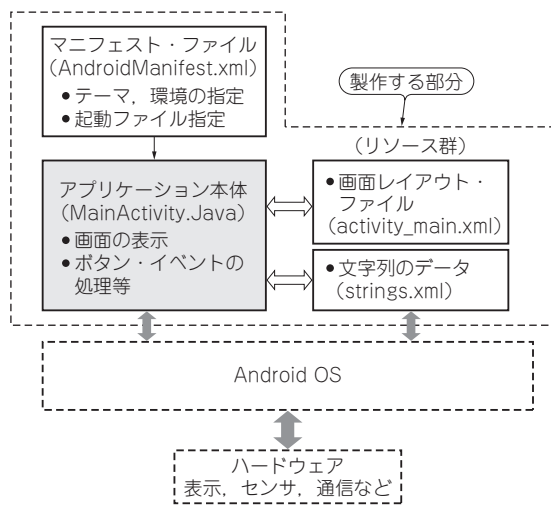
図1 製作したAndroidアプリケーション・プログラムの全体像
