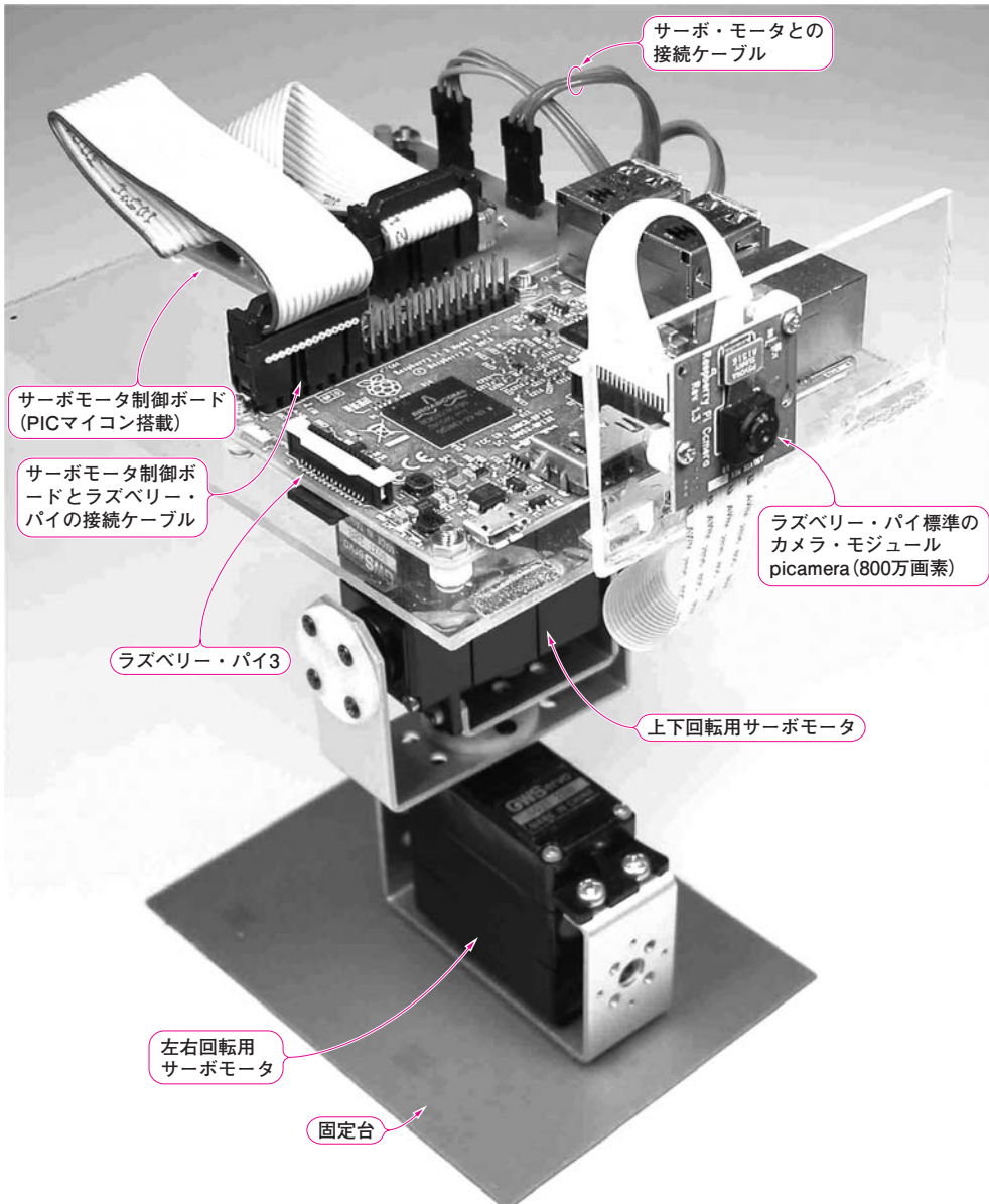
写真1 第1章～第9章の知識をフル活用! スマホでリモート制御できるロボット・ムービを製作する
