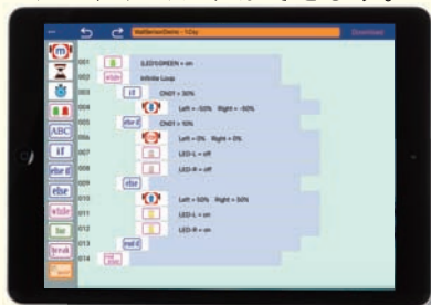
C-Style のイメージ画面
